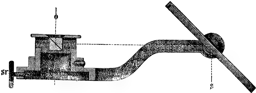
Фиг. 15. Камера люцида по Аббе, въ естеств. велич. Идеальный продольный разрѣзъ. Направленіе лучей обозначено линиями. o — направленіе, по которому смотритъ глазъ наблюдателя. s — направленіе, перпендикулярное къ поверхности рисовальной бумаги. sr — винтъ.
